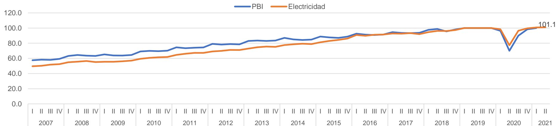
Perú: índice del PBI y demanda de electricidad desestacionalizados (2019=100)
